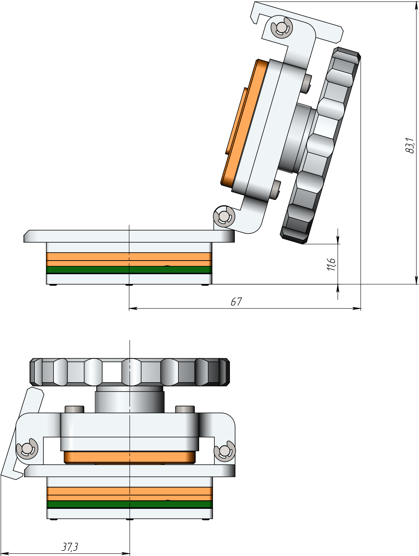
Внешний вид и габаритные размеры КУ
