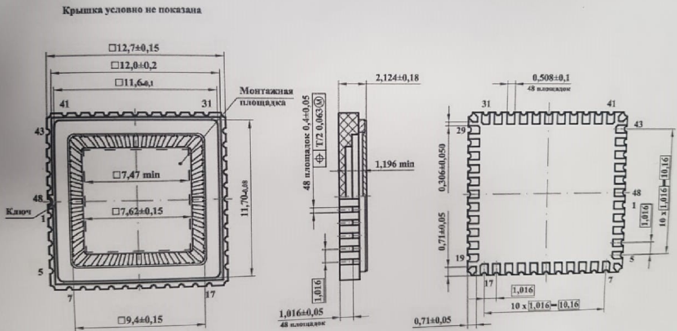
Корпус 5142.48-A
