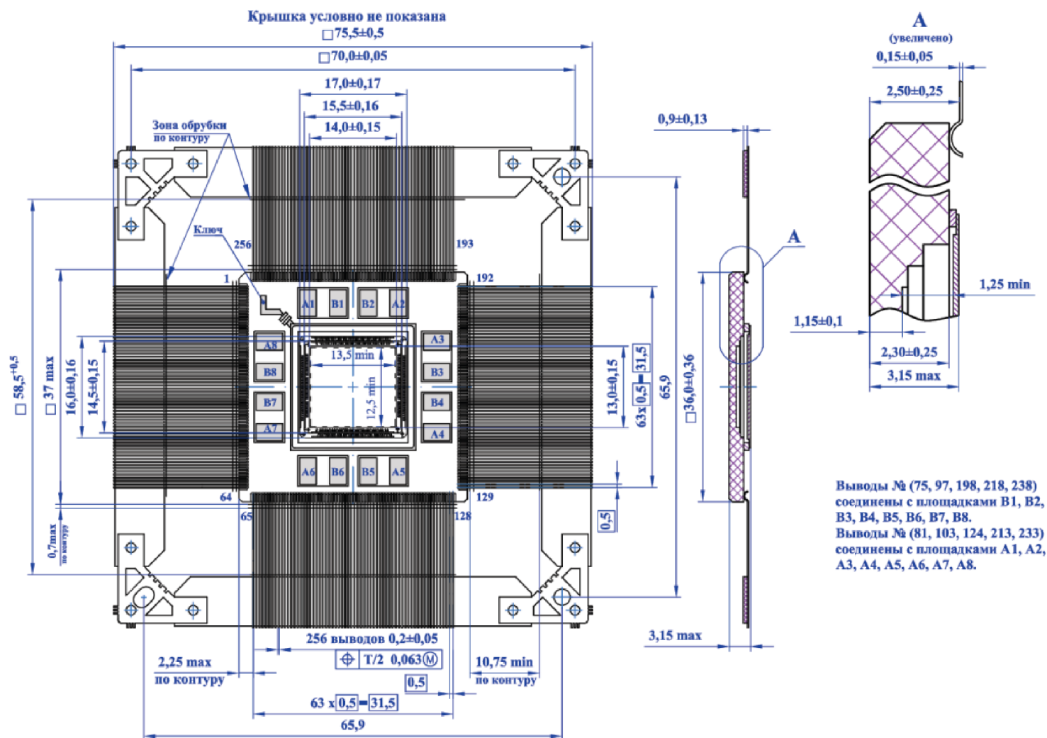
Рисунок 127 – Микросхема в корпусе 4244.256-3
