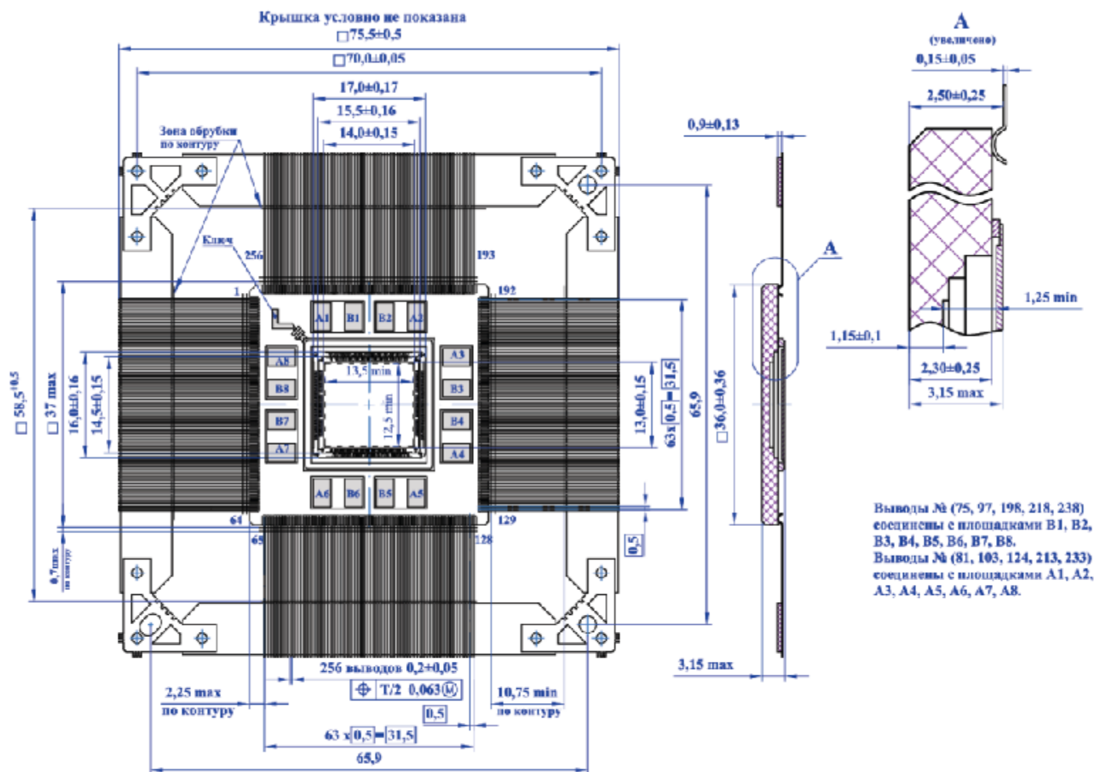
Рисунок 127 – Микросхема в корпусе 4244.256-3
