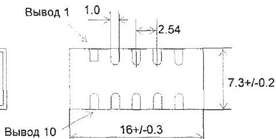
Вид снизу
