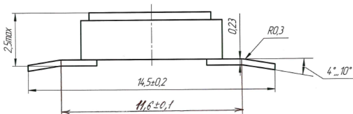
Микросхема 1127 КН61Т
