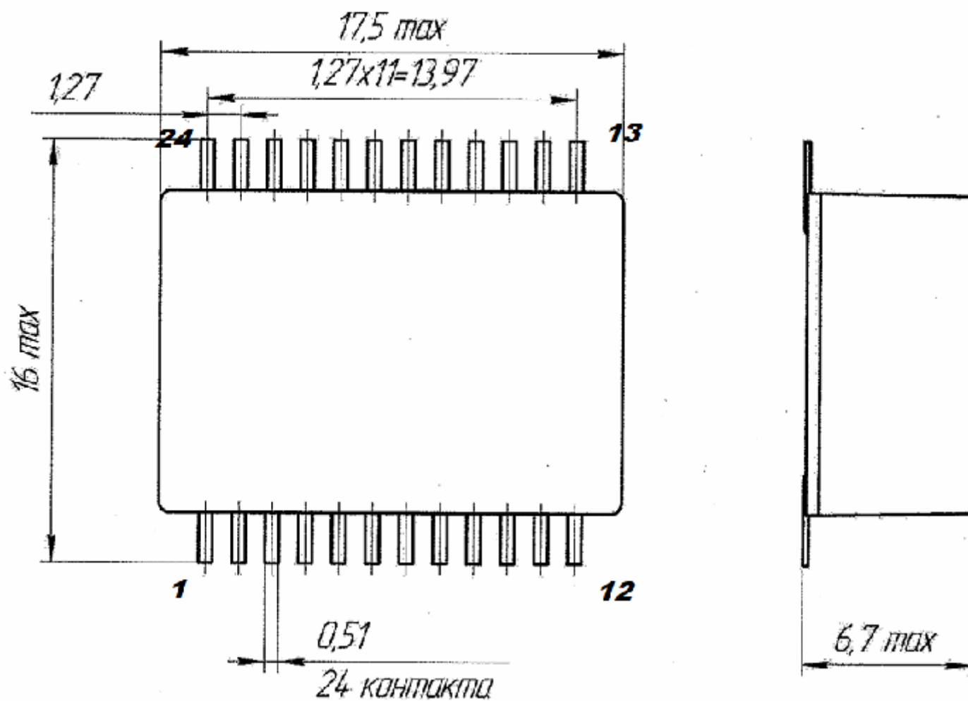
Габариты чертеж изделия
