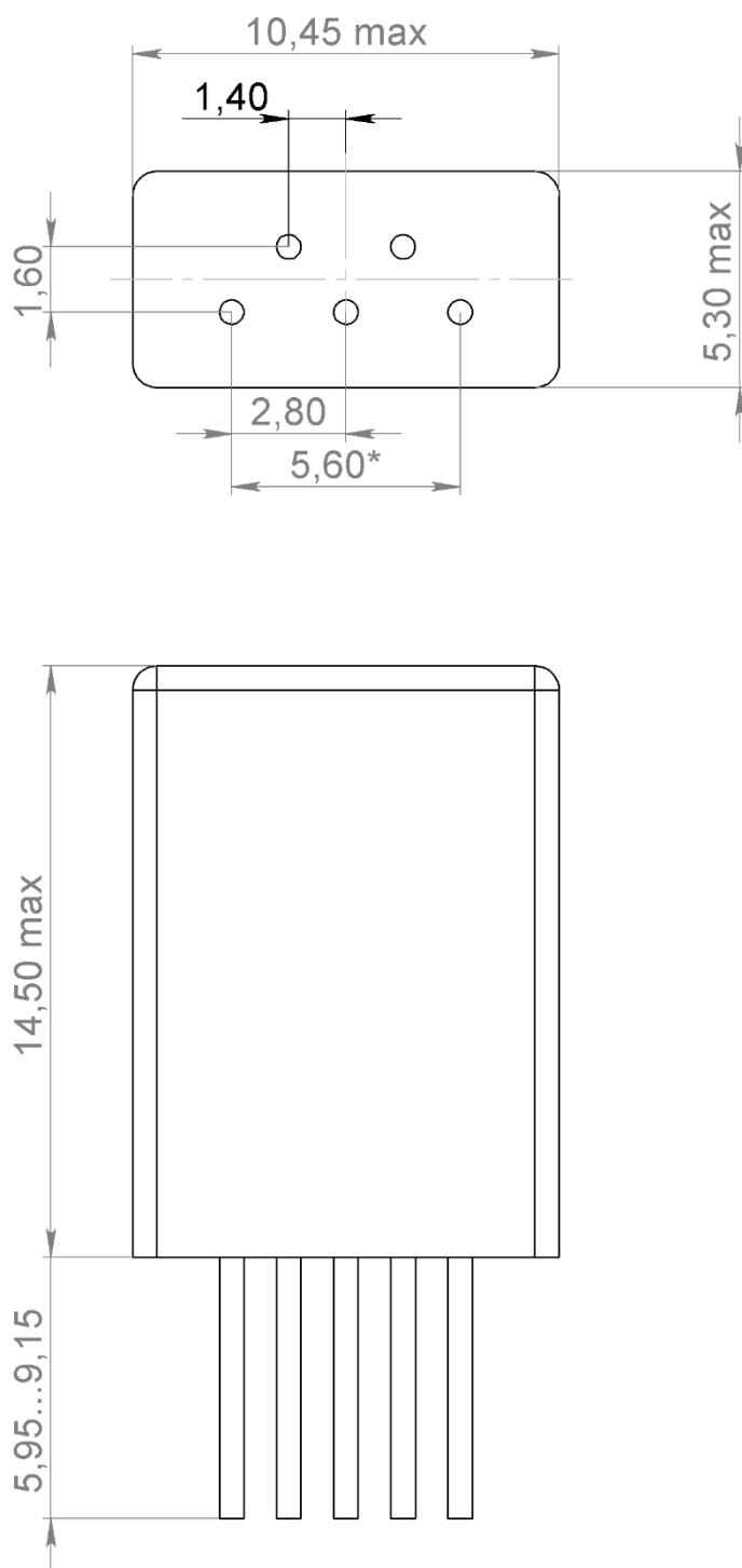
Рис. 4. Внешний вид и габариты ЭРИ (предоставляется заказчиком)
