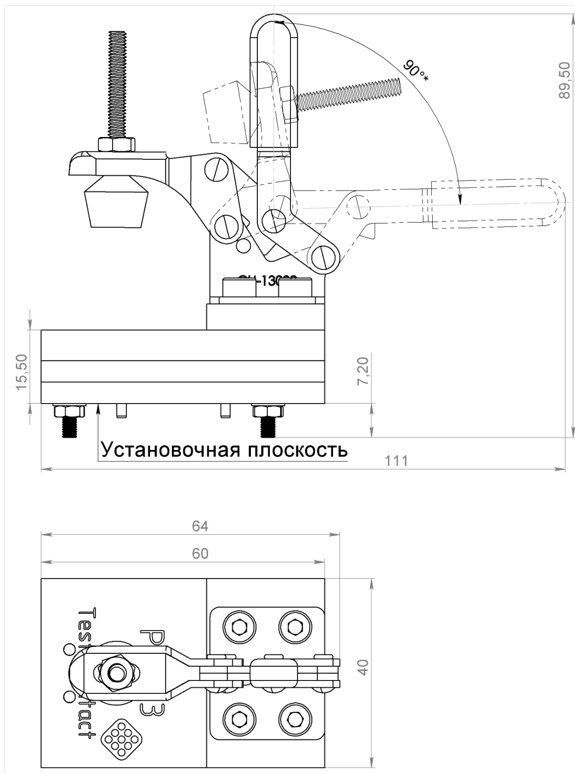
Рис. 1. Разнесенный вид КУ (контакты КУ (пины) и тестируемое изделие (ЭРИ) условно не показаны).
