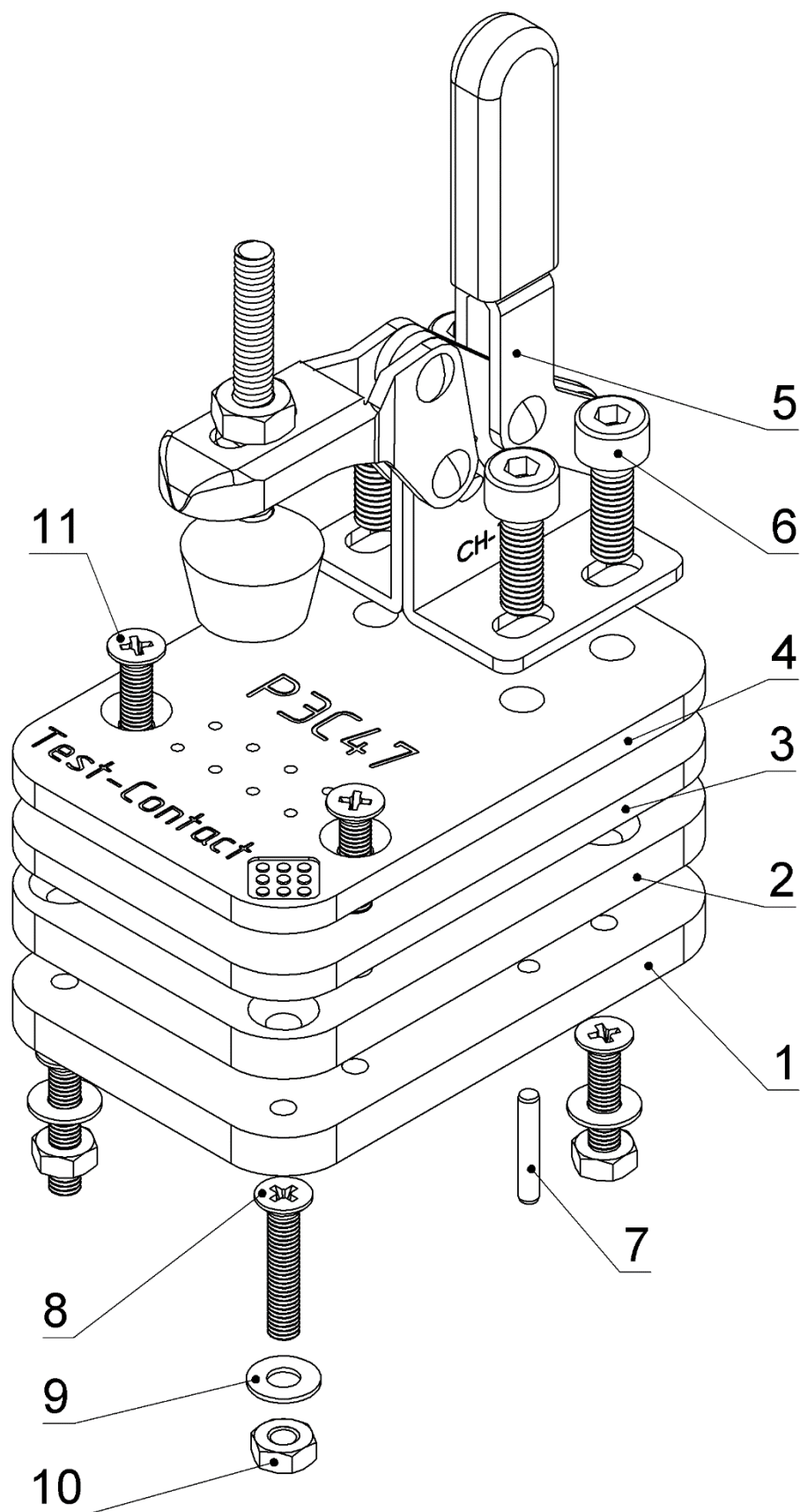
Рис. 1. Разнесенный вид КУ (контакты КУ (пины) и тестируемое изделие (ЭРИ) условно не показаны).
