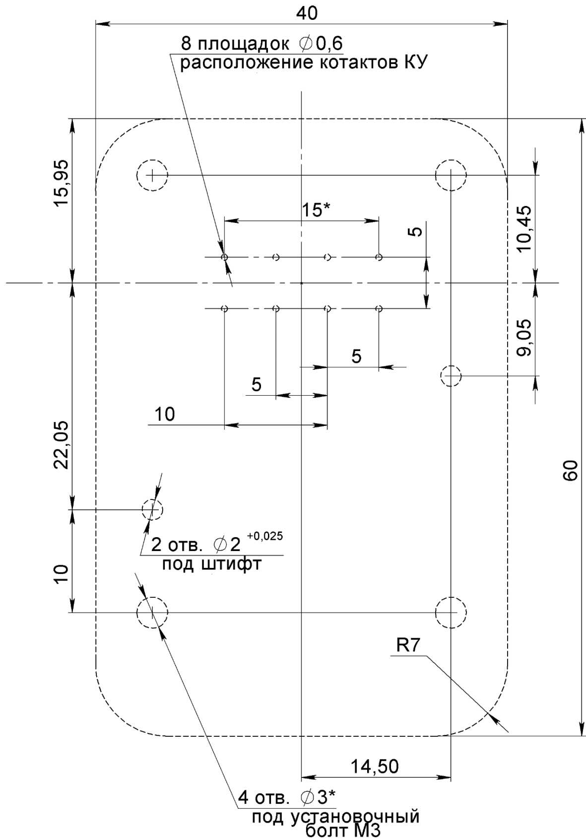
Рис. 3. Эскиз посадочного места КУ на ПП (вид на устройство сверху).
