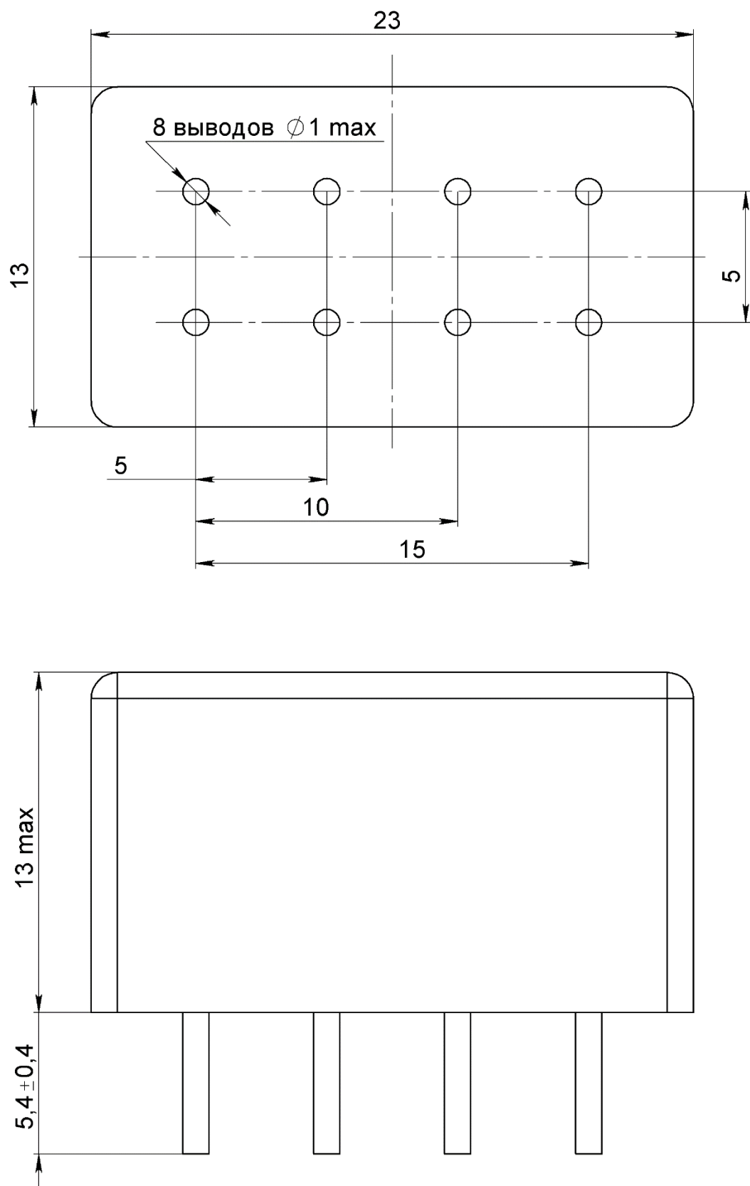
Рис. 4. Внешний вид и габариты ЭРИ (предоставляется заказчиком)
