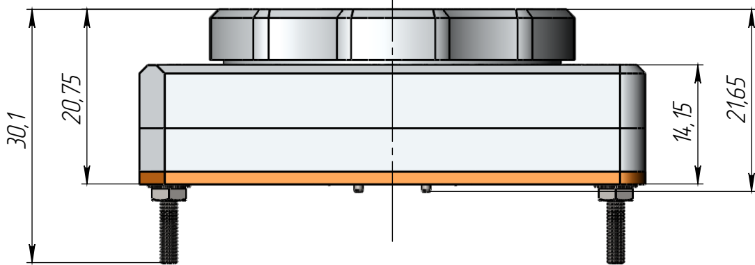
Внешний вид и габаритные размеры КУ SOP-tl-h-40-0.5-001
